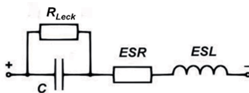
Abb. 2: Ersatzschaltbild des Elektrolytkondensators
