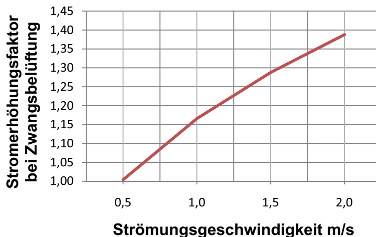
Abb. 5: Erhöhung der Strombelastbarkeit durch Zwangskühlung
