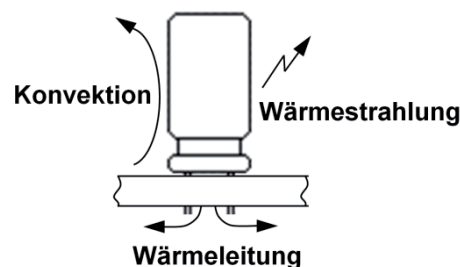
Abb. 4: Kühlungsmechanismen von Elkos
