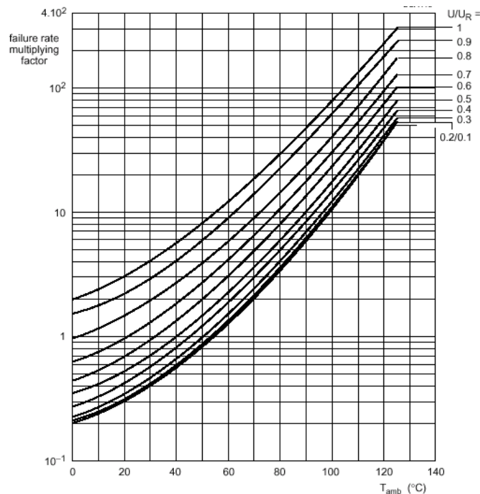
Abb. 5: Korrekturfaktoren gemäß MIL HDBK-217F
